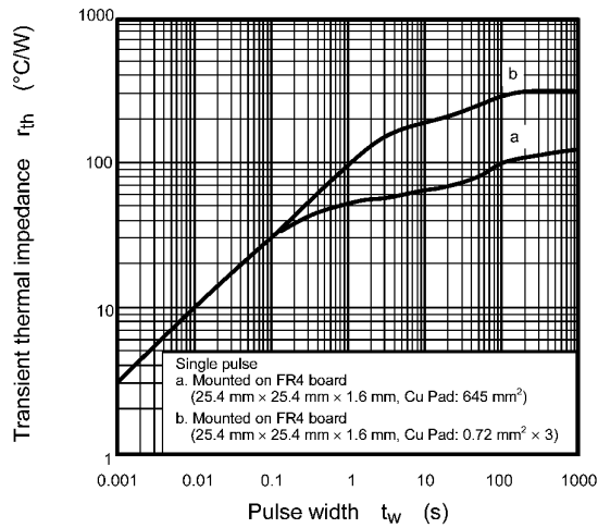
Fig. 7.13 r_{th} - t_w
